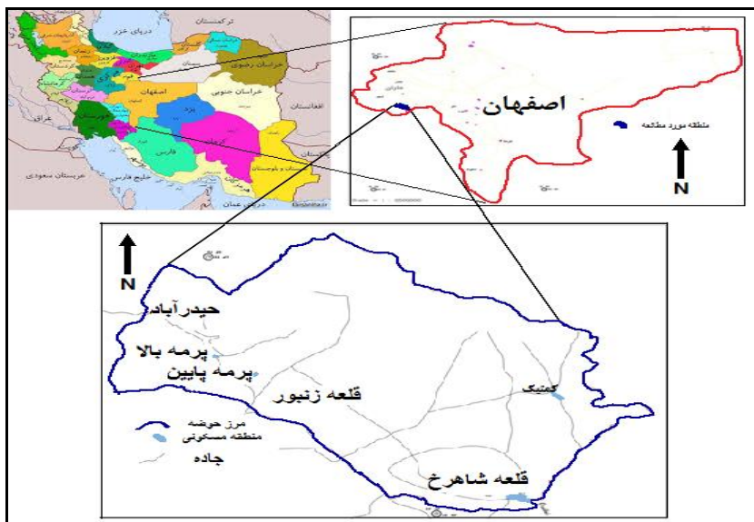
شکل ۱. نقشه موقعیت حوضه آبخیز قلعہ شاهرخ چادگان در استان اصفهان
